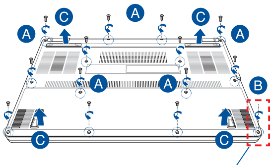
Vijak za skočno otvaranje
